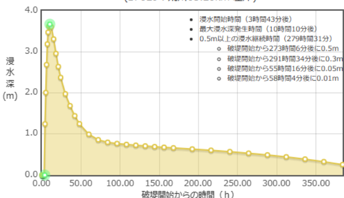
浸水シミュレーショングラフ (BP029：荒川65.20km 左岸)
